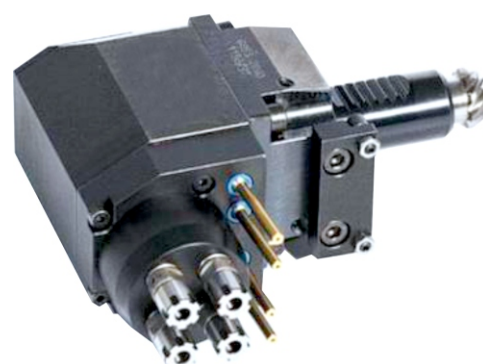
Радиальная многошпиндельная сверлильная головка
